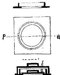
Вьюшка—видъ сверху и вертикальный разръзъ.
