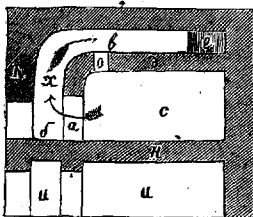
Русская печь—вертикальный продольный разрѣзъ.
