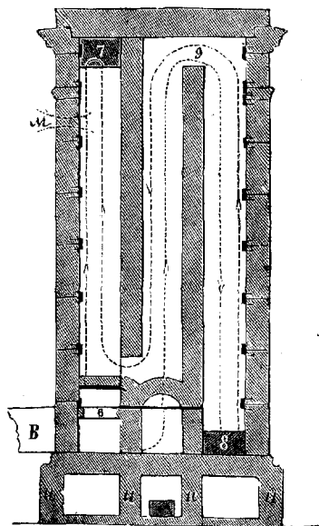
Вертикальный разръзъ голландской печи.
