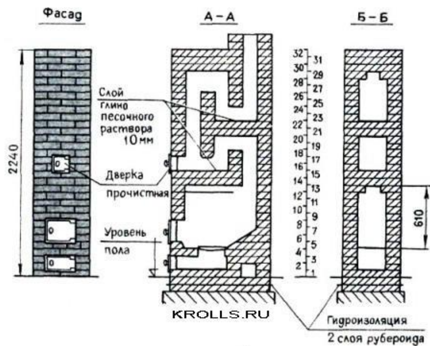
Рис. 41. Отопительная прямоугольная толстостенная печь с преимущественно нижним обогревом конструкции В. И. Стержнева (печь ПТОУ-2500)
