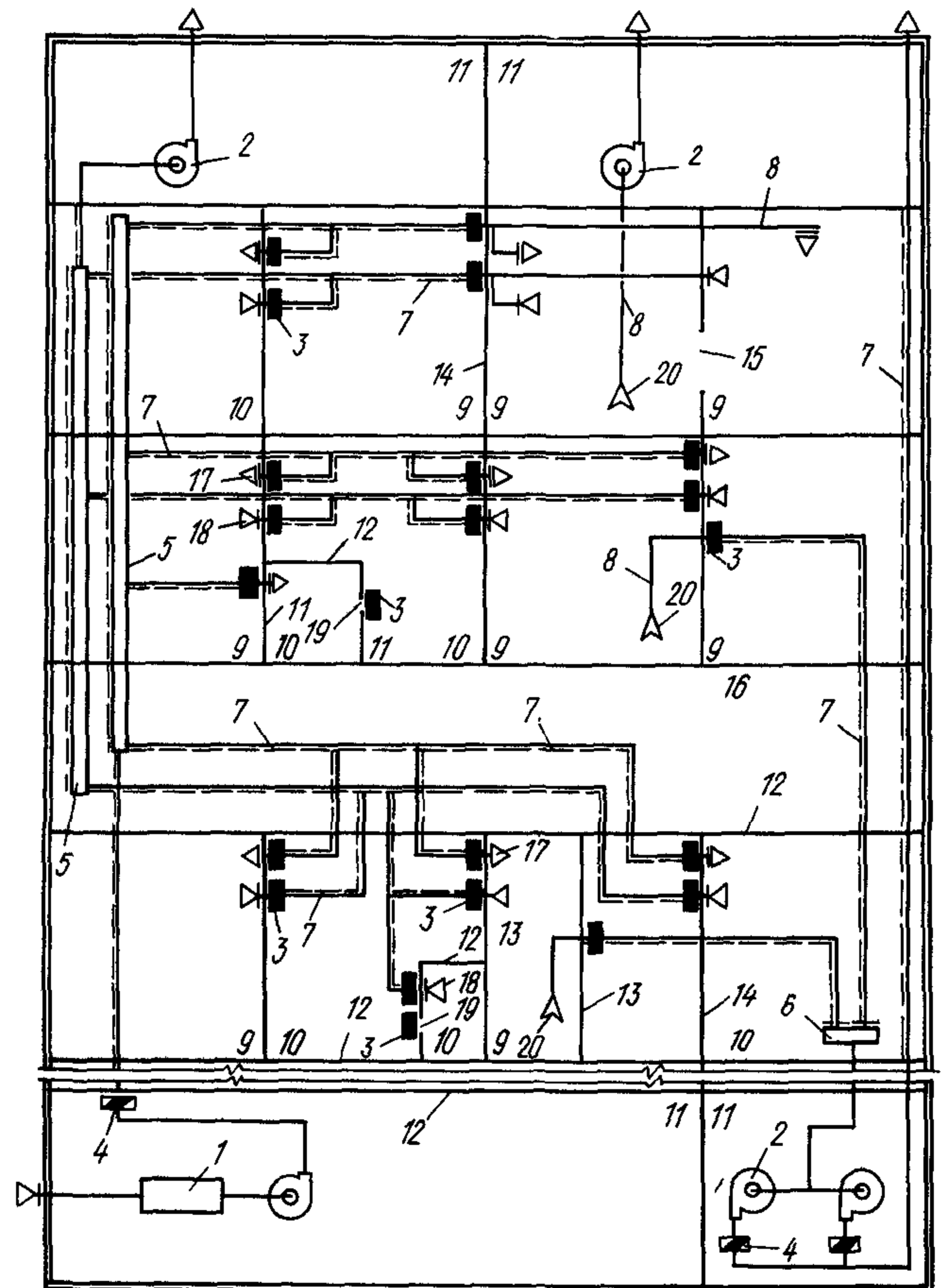
Черт. 3. Схема воздуховодов с огнезадерживающими клапанами
