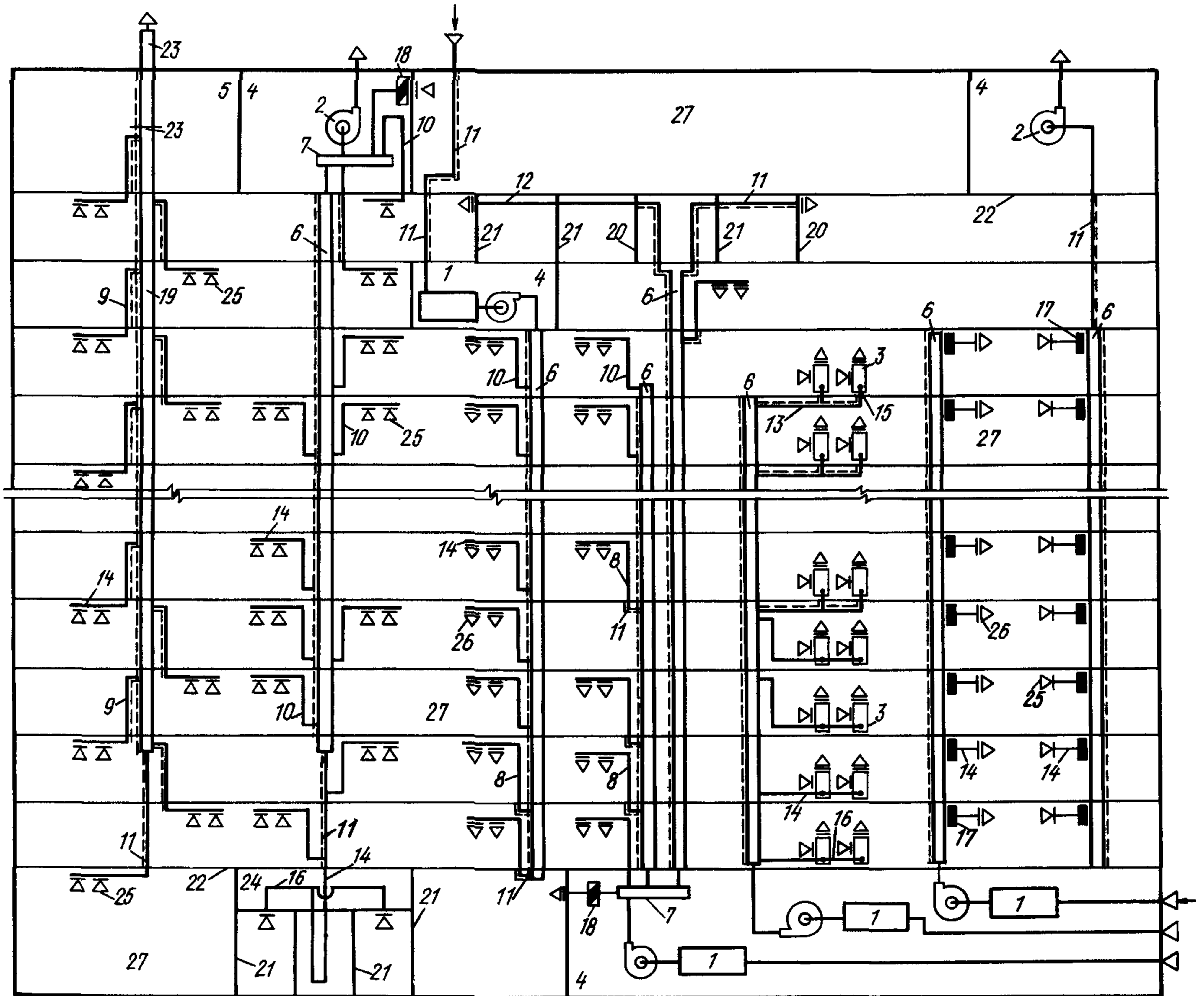
Черт. 1. Схемы воздуховодов с вертикальными коллекторами
