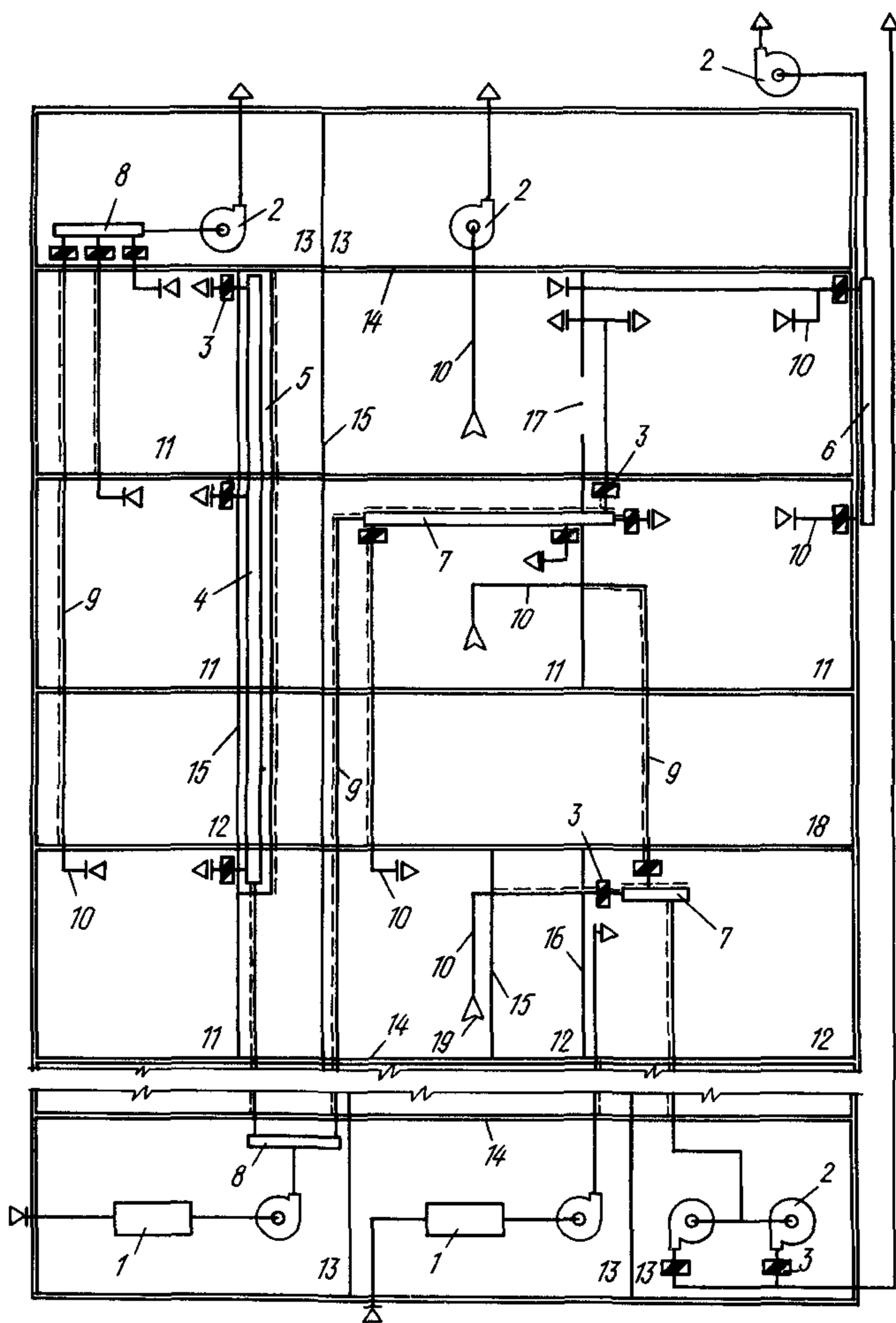
Черт. 4. Схема воздуховодов с обратными клапанами
