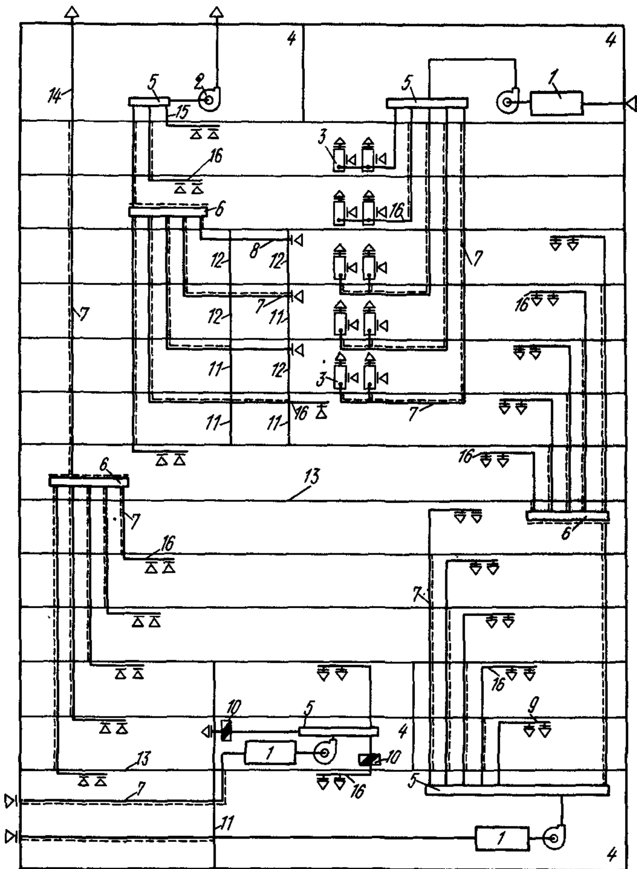
Черт. 2. Схема воздуховодов с горизонтальными коллекторами
