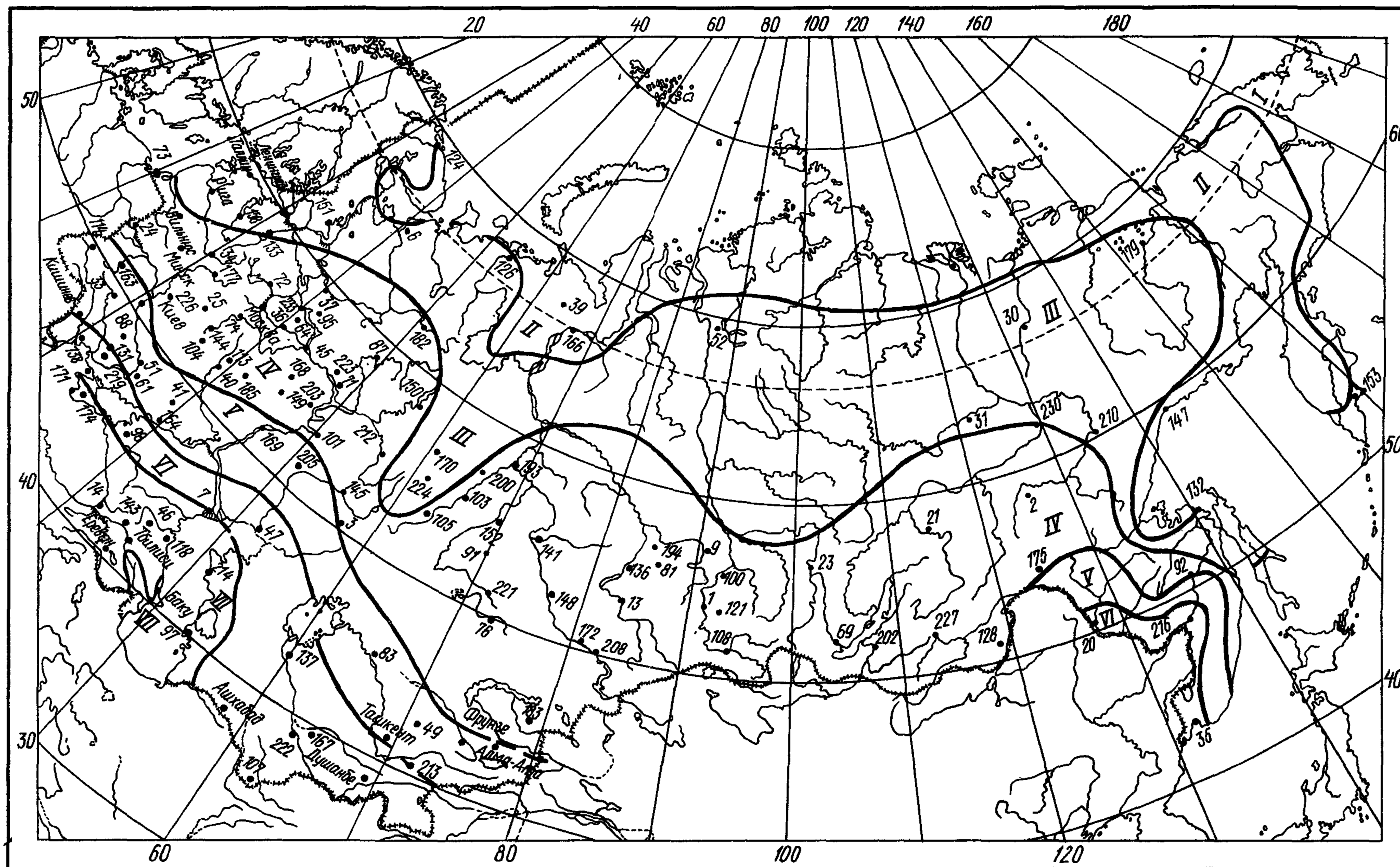
Черт. 1. Карта-схема 1 районирования территории СССР по величине удельной энтальпии I , кДж/кг, наружного воздуха в теплый период года (параметры А) для районов: I - I \leq 40 ; II - I = 40 - 43,6 ; III - I = 43,6 - 48,4 ; IV - I = 48,4 - 52,6 ; V - I = 52,6 - 56,8 ; VI - I = 56,8 - 61 ; VII - I = 61 - 65 Номер населенного пункта на карте-схеме соответствует порядковому номеру таблицы обязательного приложения 7
