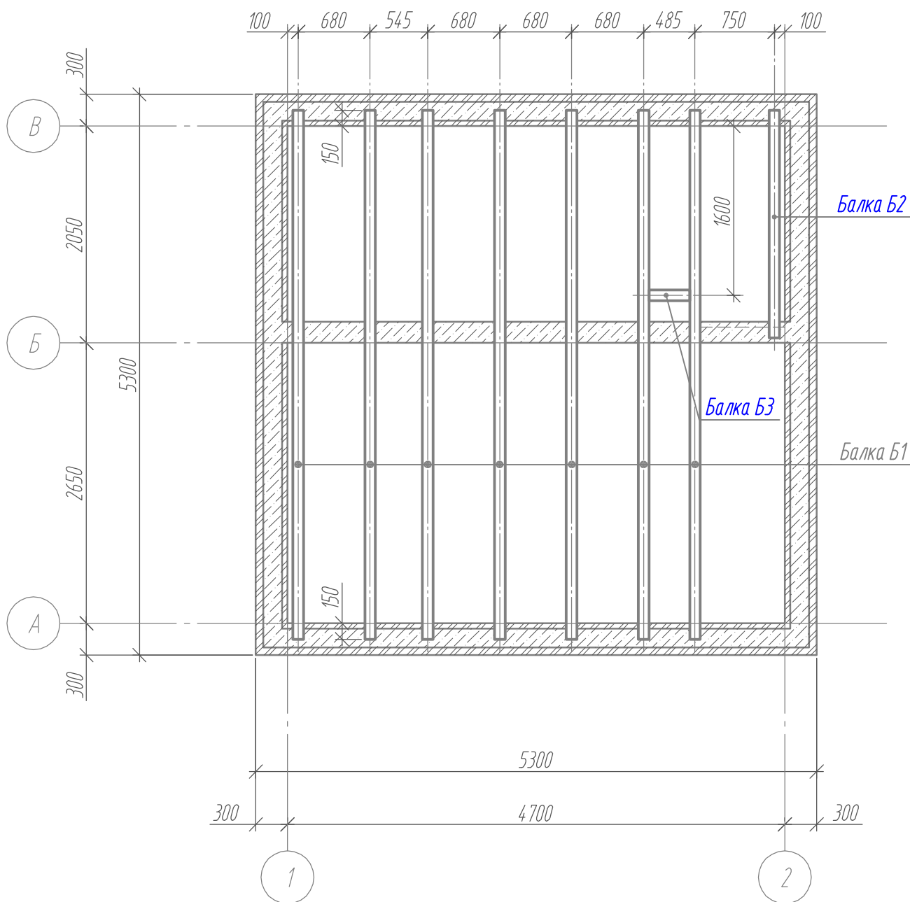
Схема расположения балок перекрытия на отм. +2,680
