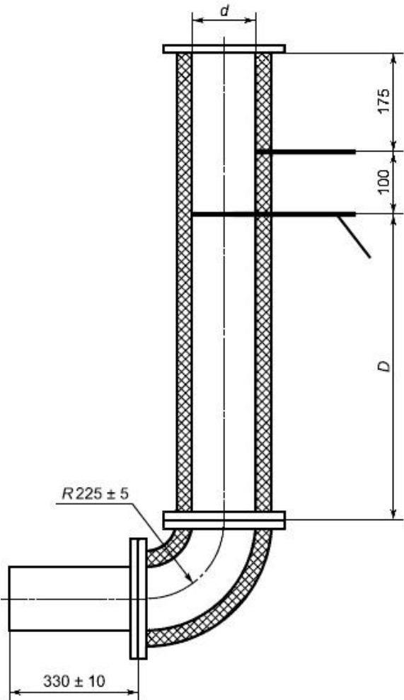
Рисунок А.10 - Детали и размеры измерительного участка для горизонтального подключения
