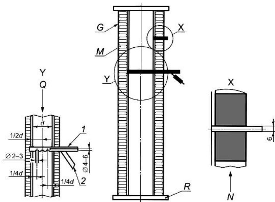
Рисунок А.8 - Конструкция и общая схема измерительного участка
