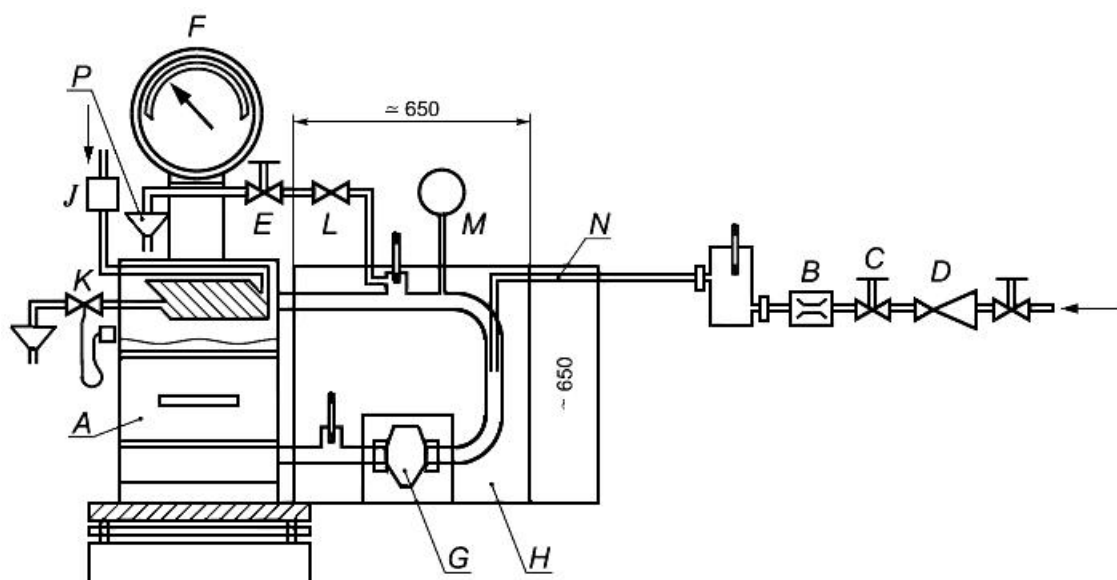
Рисунок А.11 - Пример испытательного стенда для котлов с водяным контуром
