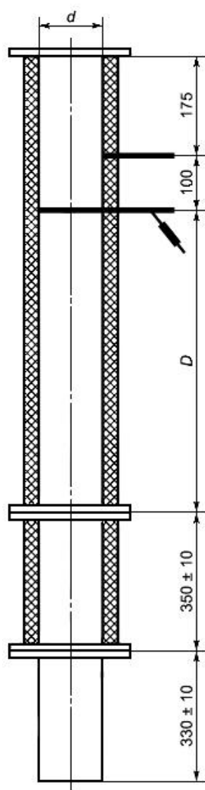
Рисунок А.9 - Детали и размеры измерительного участка для подключения вертикального дымохода
