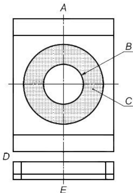
Рисунок А.4 - Деталь вставки для задней стенки испытательного угла
