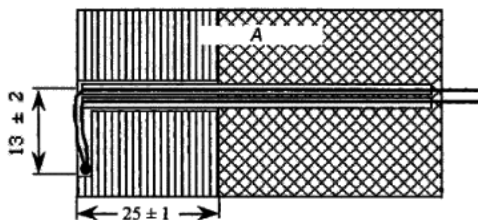
А— Стенка испытательного угла
