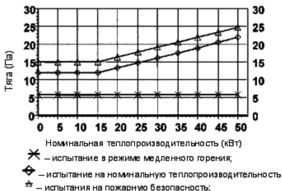
Рисунок 1 — Значения тяги в дымоходе
