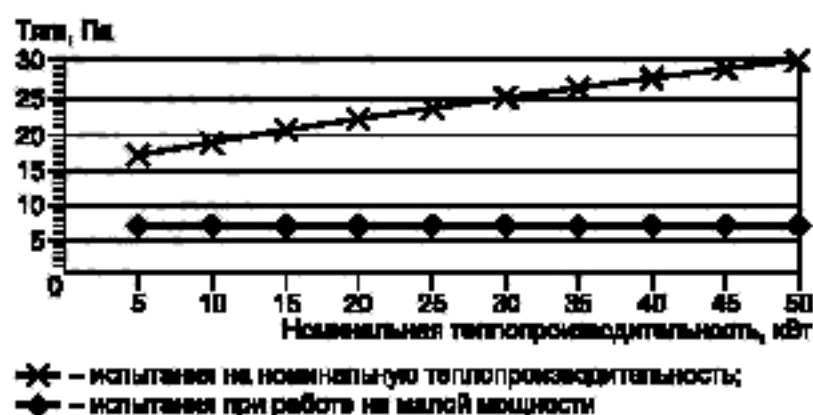
Рисунок 2 — Значения тяги в дымоходе
