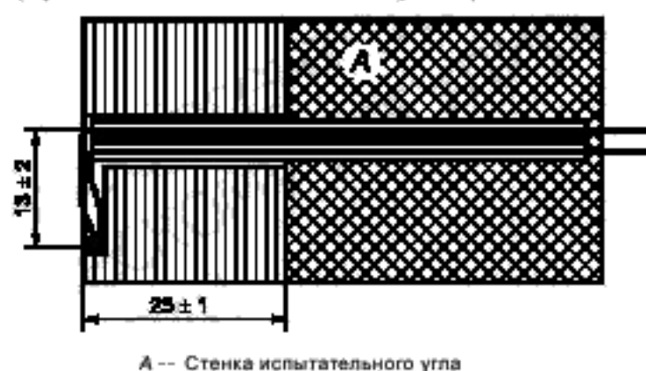
Рисунок А.7 — Расположение термозлемента в стенке испытательного угла
