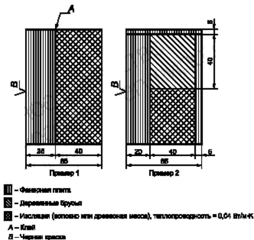
Рисунок А.5 — Разрез конструкции испытательного угла
