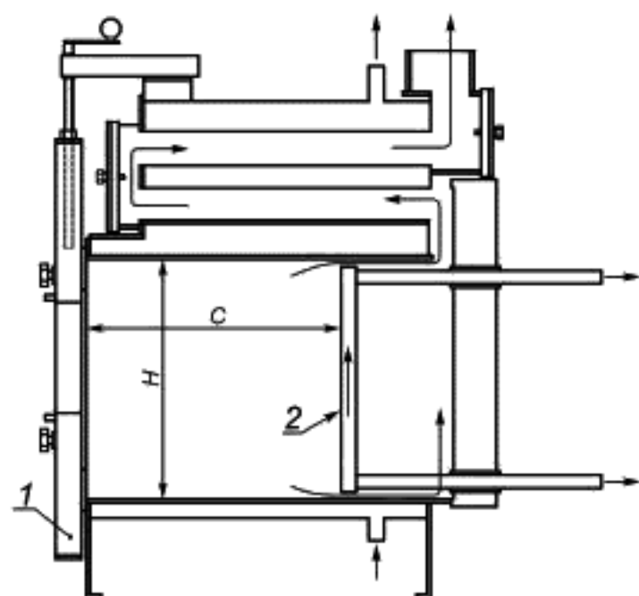
а) Вид сбоку, схема прохода
